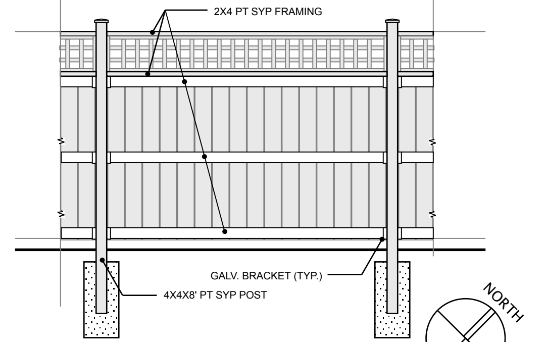
INTERIOR SIDE - SCALE: 1/2"=1'0"
