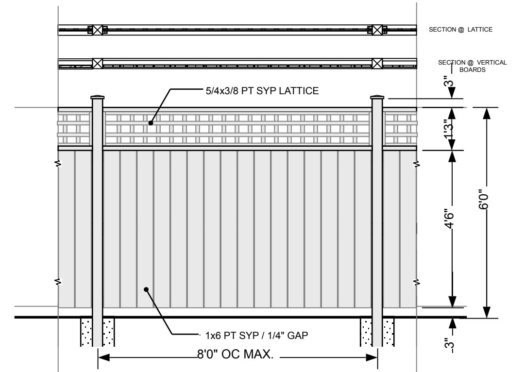
EXTERIOR SIDE - SCALE: 1/2"=1'0"
